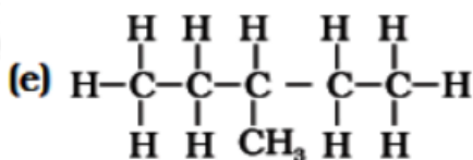
3- ميثيل بنتان
