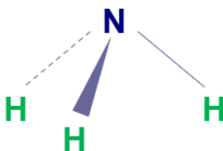
الأمونيا
