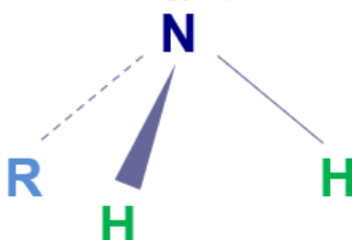
أمين أولي
