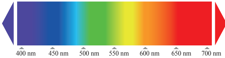
الشكل (6): الأشعة المرئية (الضوء المرئي).
