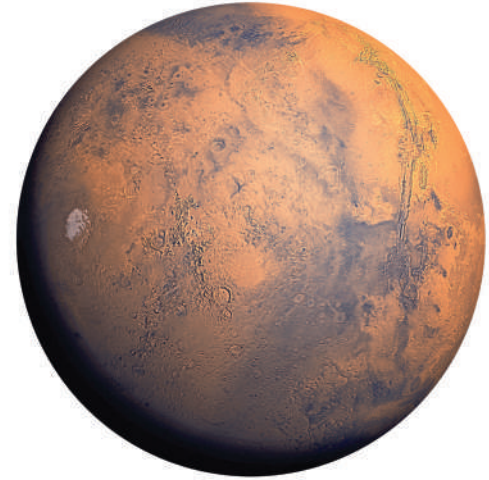
الشكل (8): كوكب المريخ.
