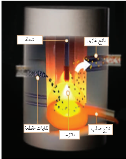
محوّل النفايات البلازمي.
