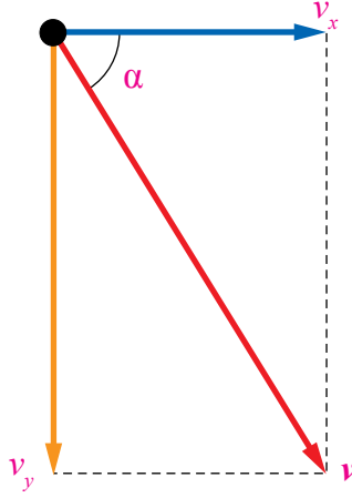
الشكل (15): اتجاه السرعة.
