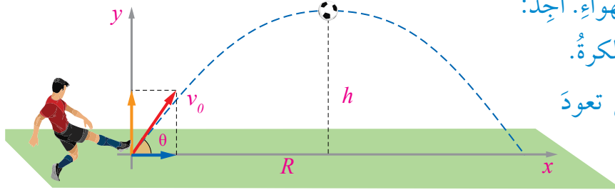
الشكل (12): مسار حركة الكرة.
