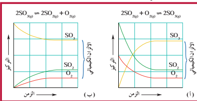
شكل (40) توضح هذه المنحنيات الباقية تغير تركيزات كل من \text{SO}_2 و \text{O}_2 مع مرور الوقت. في بداية التفاعل، يكون تركيز \text{SO}_2 صافياً تركيز \text{O}_2 مع غياب غاز \text{SO}_3 . وعند الاتزان، يتكون خليط من الغازات الثلاثة متجانسة. (ب) لا يظهر في البداية سوى غاز \text{SO}_3 . وعند الاتزان، نجد أن تركيزات \text{SO}_2 و \text{O}_2 هي نفسها الموضحة في الرسم الباقى (أ) في حالة الاتزان.
