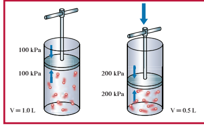
شكل (9) عندما يندفع الكباس المستخدم في المحركات بقوة إلى أسفل ، يضغط الغاز في حجم أصغر . يؤدي تقلص الحجم إلى النصف عند درجة حرارة ثابتة إلى مضاعفة الضغط الذي يمارسه الغاز .
