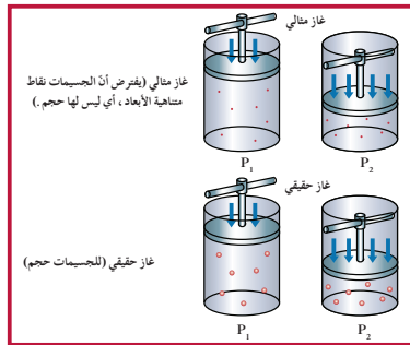
شكل (24) يجب أن يؤخذ الحجم الفعلي لجسيمات الغاز المفردة في الاعتبار كلما زاد الضغط. يصبح من الصعب ضغط الغاز بعد درجة أو نقطة معينة، مهما كانت قيمة الضغط الواقع على الغاز.
