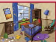
شكل (46) تكون قيمة الإنتروبي منخفضة للغرفة المرتبة التي تمّ تنظيفها حديثاً، ولكن الغرفة تصبح غير مرتبة وغير منظّمة مع مرور الوقت فتميل قيمة الإنتروبي إلى الارتفاع. ويعمل قانون الفوضى أيضاً على مستوى الذرّات والجزيئات فيمكن تطبيق المبدأ نفسه على المستوى الذري والجزيئي.
