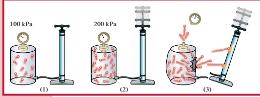
شكل (6) عندما يُضخّ غاز في وعاء قوي مغلق عند درجة حرارة ثابتة، يزداد الضغط بنسبة عدد جسيمات الغاز المضاعفة. وكذلك تضاعف عدد جسيمات الغاز تضاعف الضغط. والعكس صحيح، فإذا سُمح للهواء بالخروج من الإطار المطاطي يقلّ الضغط في داخله، إذ تمارس جسيمات الغاز التي قلّ عددها (نتيجة خروج الهواء) ضغطاً أقلّ.
