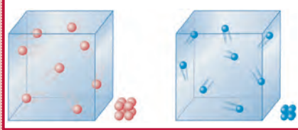
شكل (26) يسهل احتواء وعاء ما العدد نفسه من الجزيئات الكبيرة أو الصغيرة نسبياً طالما أنها ليست مترابطة بإحكام. فالفرغ كبير بالمقارنة مع الحجم الذي تشغله الجسيمات. وعندما تكون الجسيمات مترابطة بإحكام، تأخذ الجسيمات الكبيرة مساحة أكبر من الجسيمات الصغيرة.
