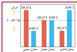
شكل (60) تركيزات كاتيون الهيدرونيوم وأنيون الهيدروكسيد في محلول حمضي ومحلّ قاعدي ومحلّ متعادل.
