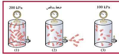
شكل (7) ضغط يتناقص عند ضغط الغاز داخل هذا الوعاء ذي الحجم الثابت عند درجة حرارة ثابتة يقلّ كلّما خرجت جسيمات الغاز (من الصورة العلوية للوعاء). عدد جسيمات الغاز عند ضغط 100 kPa هو نصف عددها عند ضغط 200 kPa.
