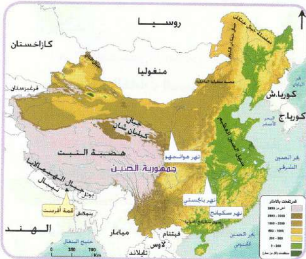
خريطة تضاريس الصين
