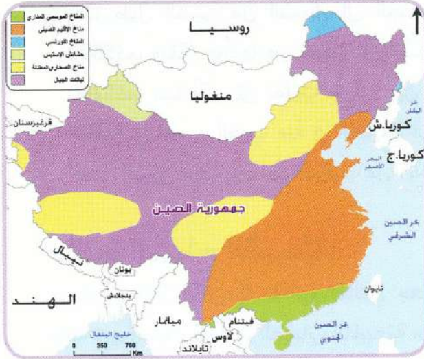
خريطة الأقاليم المناخية والنباتية
