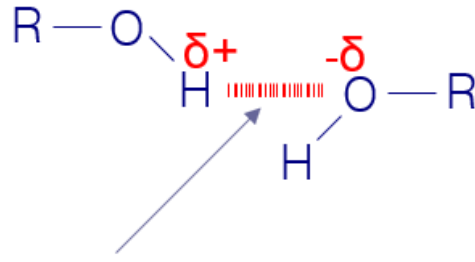
رابطة هيدروجينية
